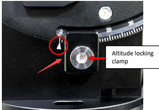
Figure 16. Setting the latitude
