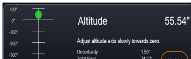
Fig. 19: Ventana de ajuste de eje de altitud durante alineación polar en CPWI.
