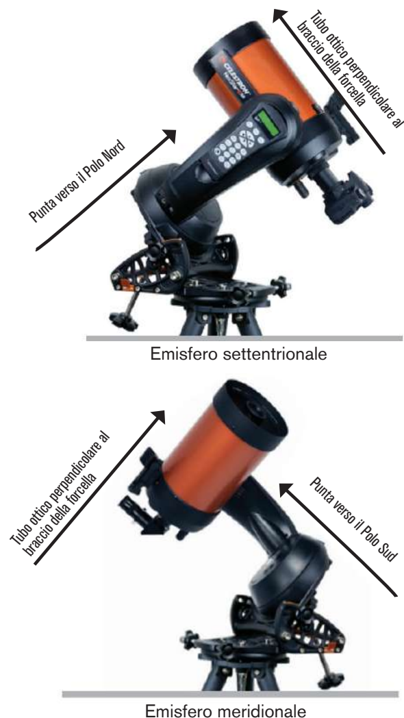
Fig. 12: Quando si utilizza una montatura a forcella altazimutale (AZ) su una base equatoriale, iniziare con la montatura nella posizione mostrata. Il braccio della forcella deve essere rivolto esattamente verso Nord (oppure verso Sud nell'emisfero australe) e il tubo ottico deve essere perpendicolare al braccio della forcella.
