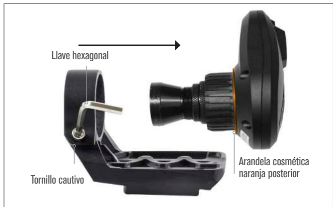
Fig. 7: Aflojar el tornillo cautivo Retirar SSAA del soporte grande, incluyendo la arandela naranja posterior.
